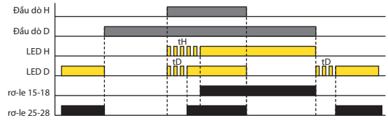
GIẾNG - TẮT TRỄ, ON DELAY (Chức năng 7)
