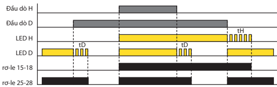
GIẾNG - TẮT TRỄ, OFF DELAY (Chức năng 7)
