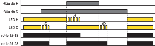
BƠM XUỐNG (PUMP DOWN), OFF DELAY (Chức năng 6)
