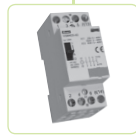
VSM425 Số lượng tiếp điểm: 4x 25 A Cấu hình của tiếp điểm chuyển đổi và ngắt: 40, 31, 22, 04.
