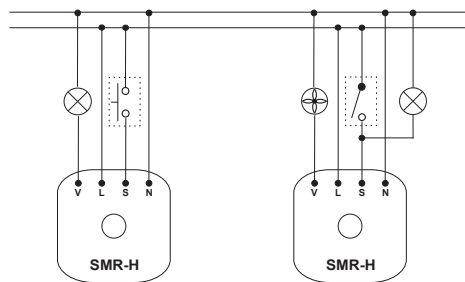
Nối dây điện hình SMR-H - bộ hẹn giờ cho quạt
