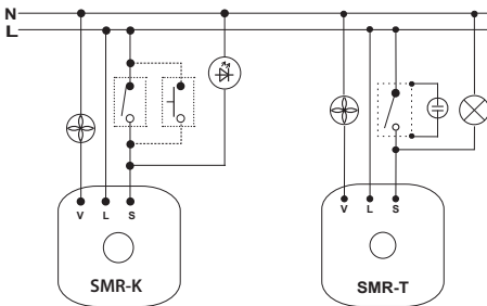
Nối dây điện hình SMR-K - bộ hẹn giờ cho quạt
