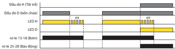
BỂ CHỨA - TẮT TRỄ, OFF DELAY (Chức năng 8)
