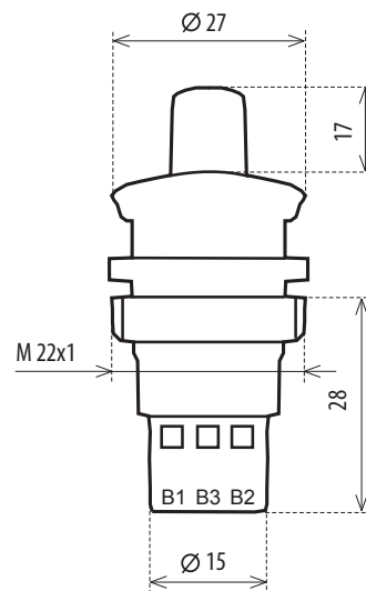
Chiết áp đơn vị điều khiển chiết áp ngoài cho CRM-91HE và CRM-2HE,
