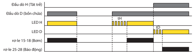
BỂ CHỨA - TẮT TRỄ, ON DELAY (Chức năng 8)
