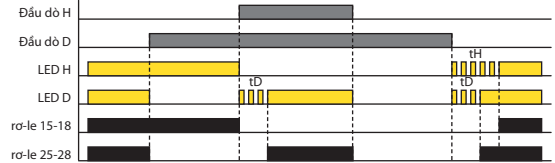
BƠM XUỐNG (PUMP DOWN), ON DELAY (Chức năng 6)
