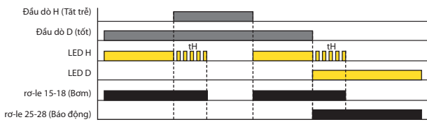
GIẾNG - TẮT TRỄ, OFF DELAY (Chức năng 7)
