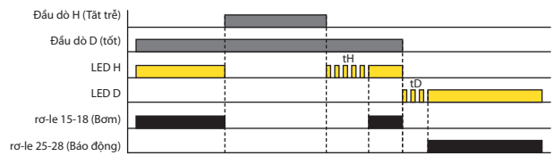
GIẾNG - TẮT TRỄ, ON DELAY (Chức năng 7)
