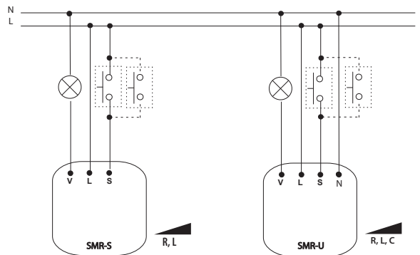
Kết nối điện hình của SMR-S - dụng cụ giảm độ sáng đèn
