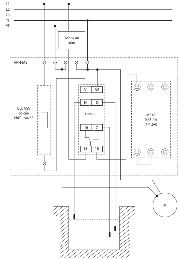
Điều chỉnh mức HRH-MS-1A (HRH-MS-1.6A)
